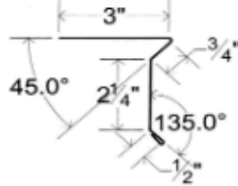
Long Drip Edge
