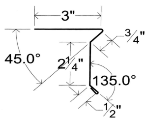
Long Drip Edge
